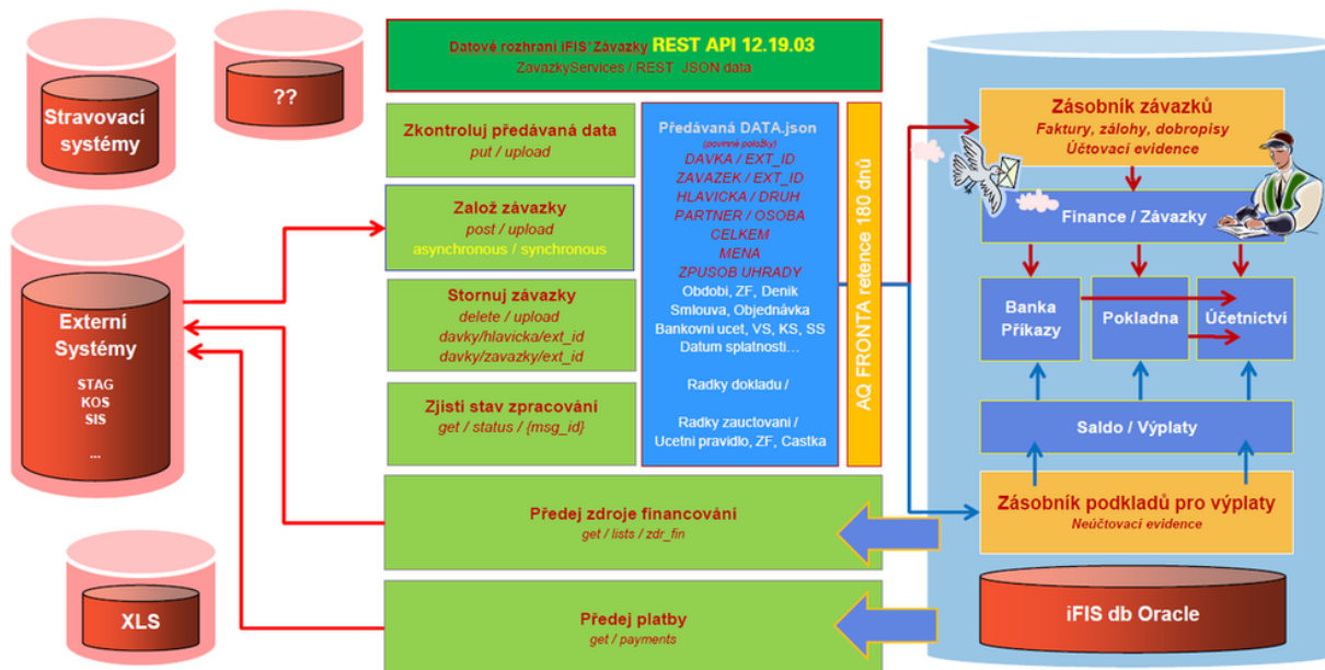
Obr. REST rozhraní iFIS Závazky - schéma
