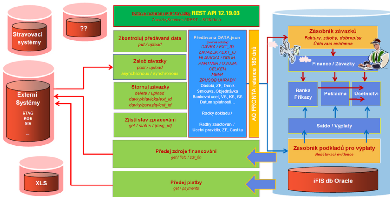
Obr. REST rozhraní iFIS*Závazky - schéma
